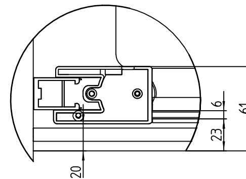
Detail Z M 1:2
