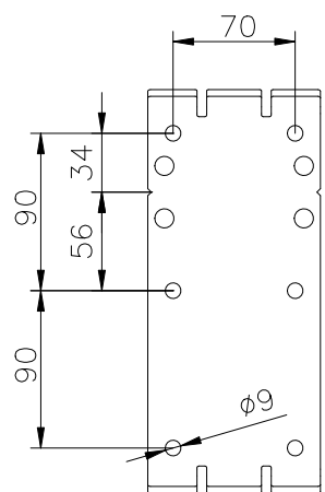
Montageskizze
